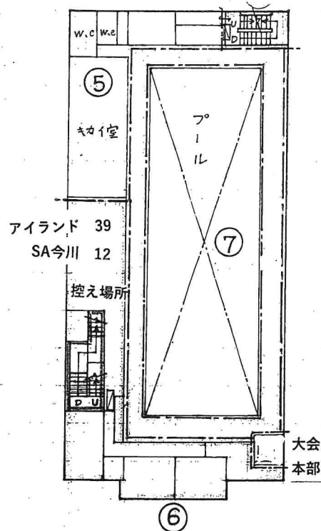
2 階設備図
